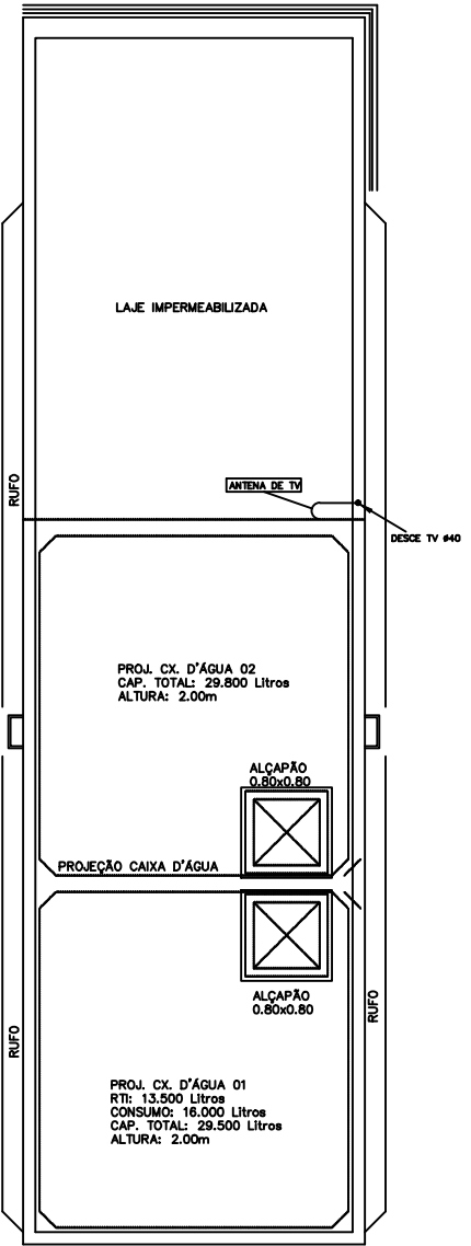
CAIXA D'ÁGUA ESCALA 1:100
