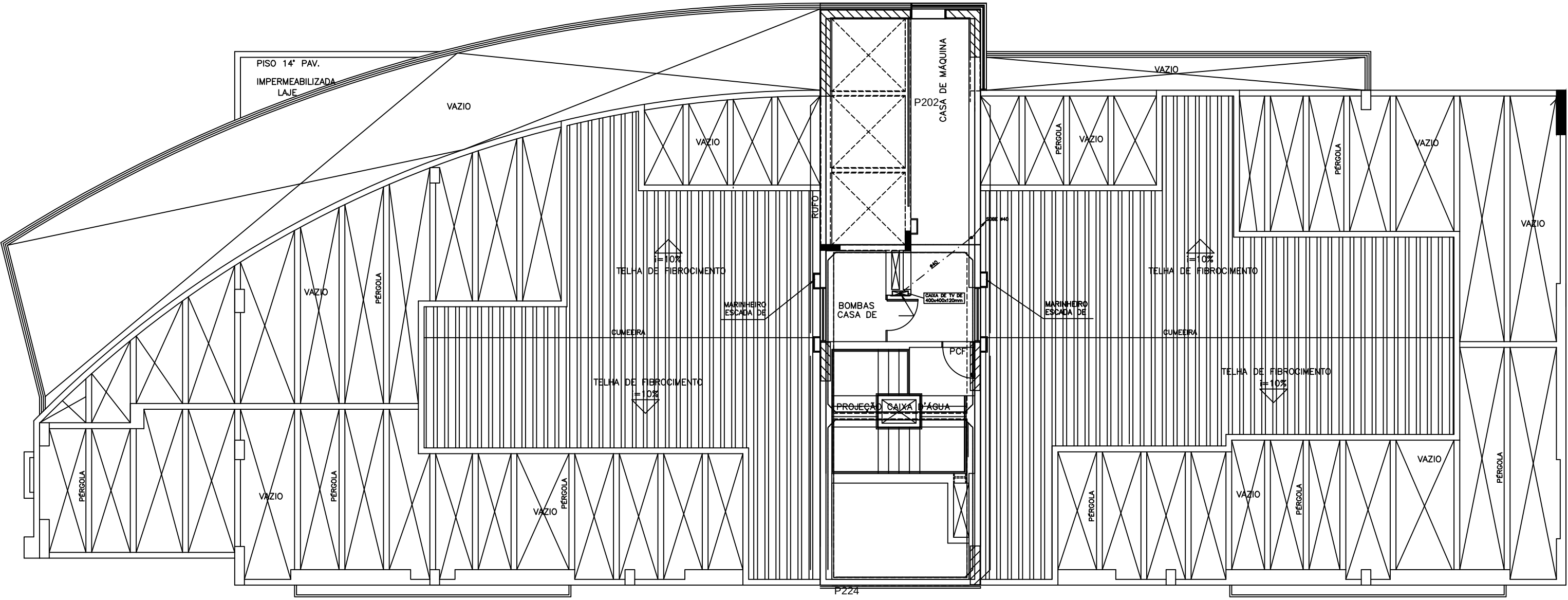
PLANTA BAIXA COBERTURA – BLOCO “B” RESIDENCIAL ESCALA 1:50
